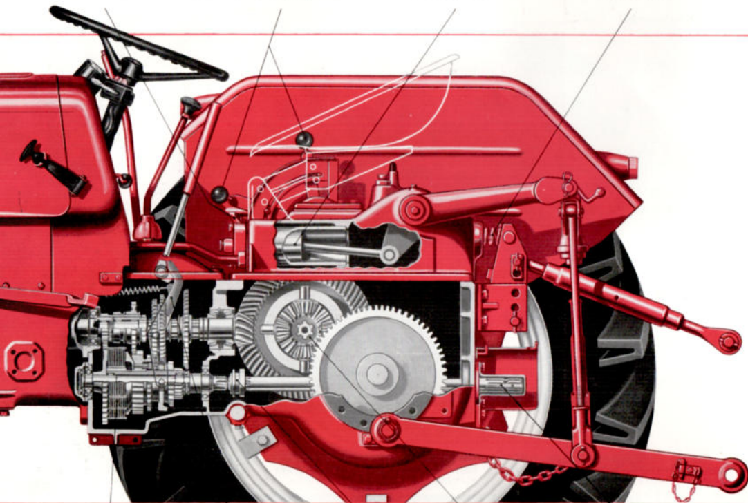
Absenkdrossel Schalthebel für Regelhydraulik Arbeitszylinder Ausgleichfeder
