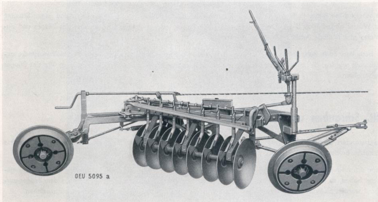
Bild 5: Pflug D 1-800 mit 8 Scheiben
