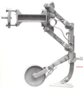
Einzel-Parallelogramm Extra 215, verlängert
