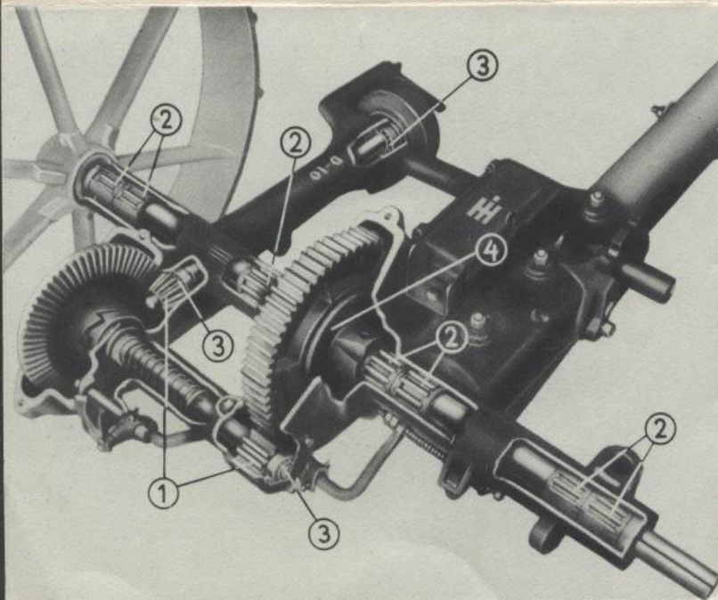
Leichtzügig und geräuschlos durch 5 Kugel- und 8 Rollenlager. Das neuartige Zweistufengetriebe läuft im Ölbad.
