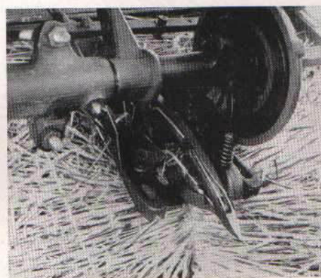
Gerade beim Knüpfvorgang ist das Bindegarn der größten Belastung ausgesetzt. Nur ein Qualitätsbindegarn garantiert störungsfreies Arbeiten.
