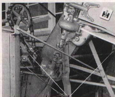
Das Bild zeigt einen Ausschnitt der Bindegarnführung am McCORMICK-Zapfwellenbinder.
