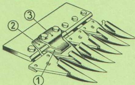
Die Messerführung DRP. 637 572 und 653 803 (1) Reinigungsplatte; (2) Reibungsplatte; (3) Messerhalter
