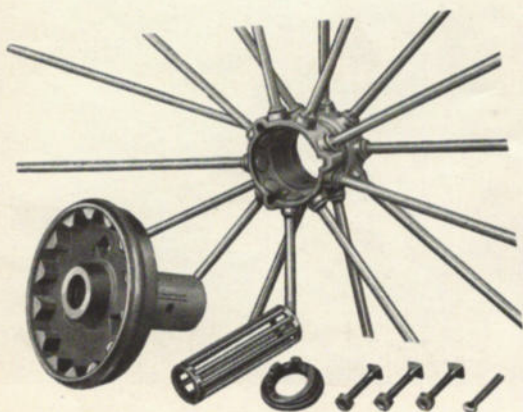
Radnabe und Sperrscheibe sind aus einem Stück und können leicht ausgewechselt werden. Rollenlager in den Fahrrädern erhöhen die Leichtzügigkeit des Gerätes.
