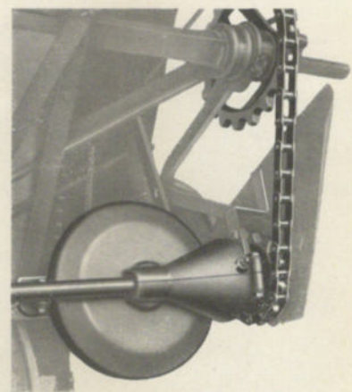
Gezapfeltes Hauptwinkelgetriebe.
