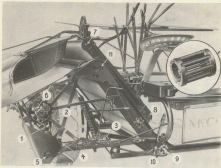
Rollenlager am M C CORMICK Bindemäher Nr. 5: 1 und 2-Haupttrad mit Kugeldrucklagern / 3 und 4-Gegenwelle mit Kugeldrucklager / 5-Kurbelwelle / 6-Binderantriebswelle / 7 und 8-Obere Elevatorwalzen / 9-Plattformwalze / 10 und 11-Untere Elevatorwalzen
