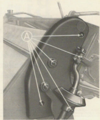
Gezapfelter Elevatorantrieb. A. Die bequeme und zuverlässige Fettpressenschmierung.
