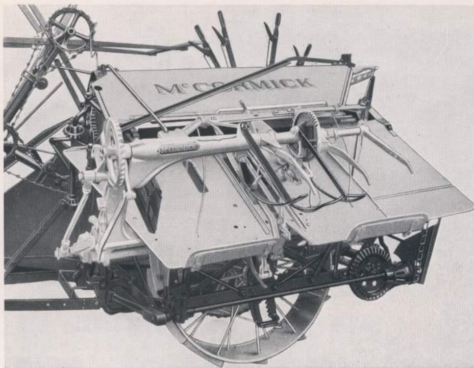
Breiter stählerner Bindetisch und langer Bindearm für längstes Getreide. 2 Garbenabstreifer.
