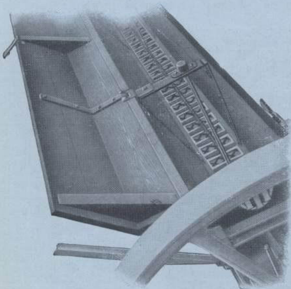
Blick in den Streukasten mit Streumechanismus
