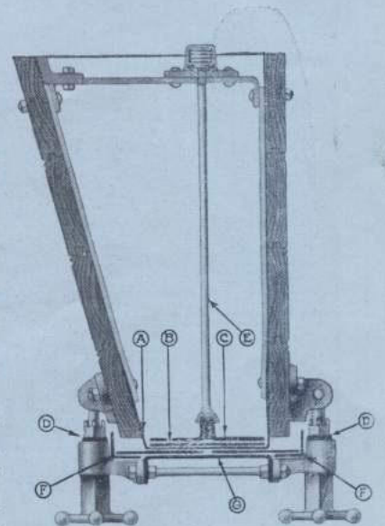
Querschnitt durch den Streukasten und Streumechanismus
