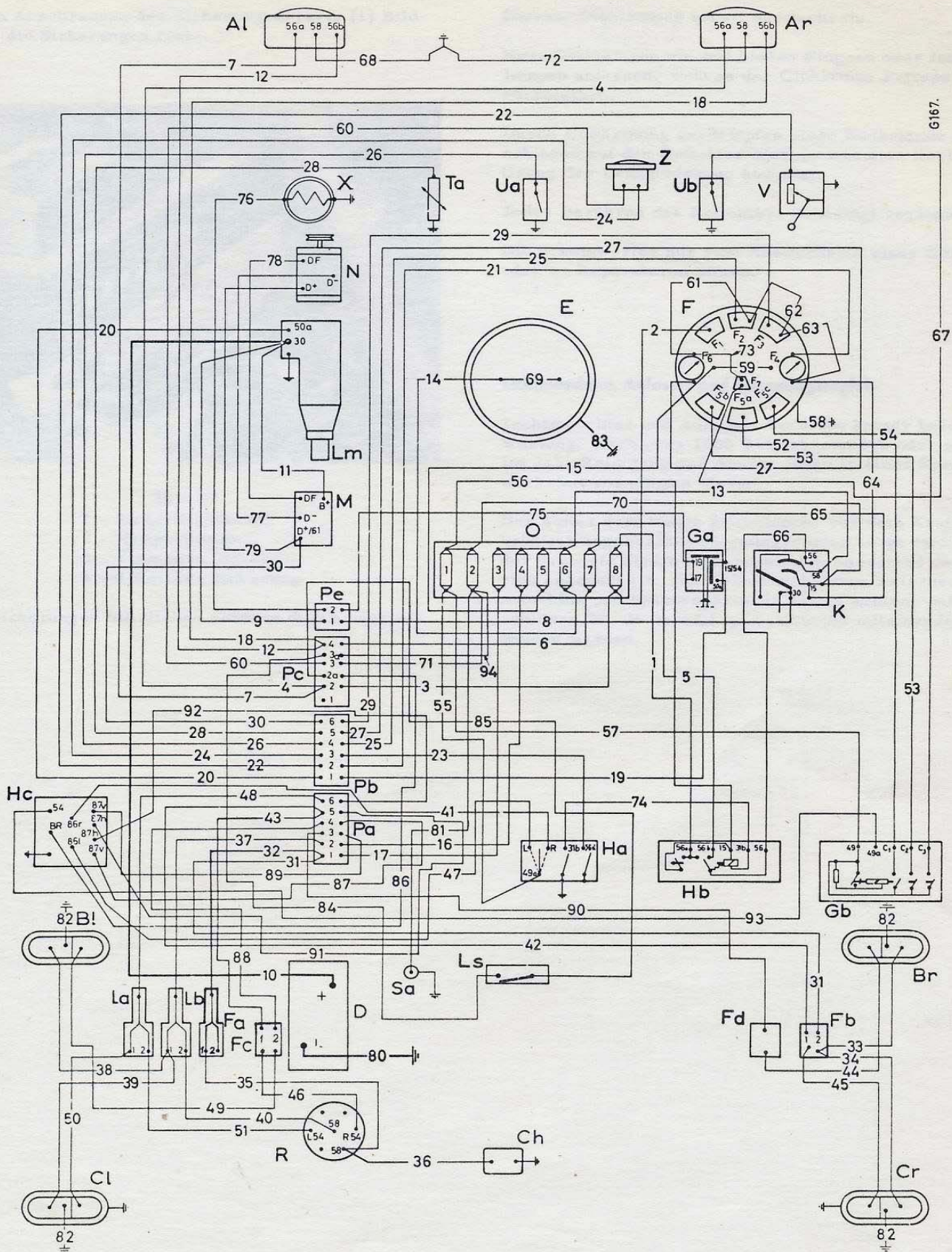
** Schaltschema für Schlepper mit Geschwindigkeiten über 20 km/std.
