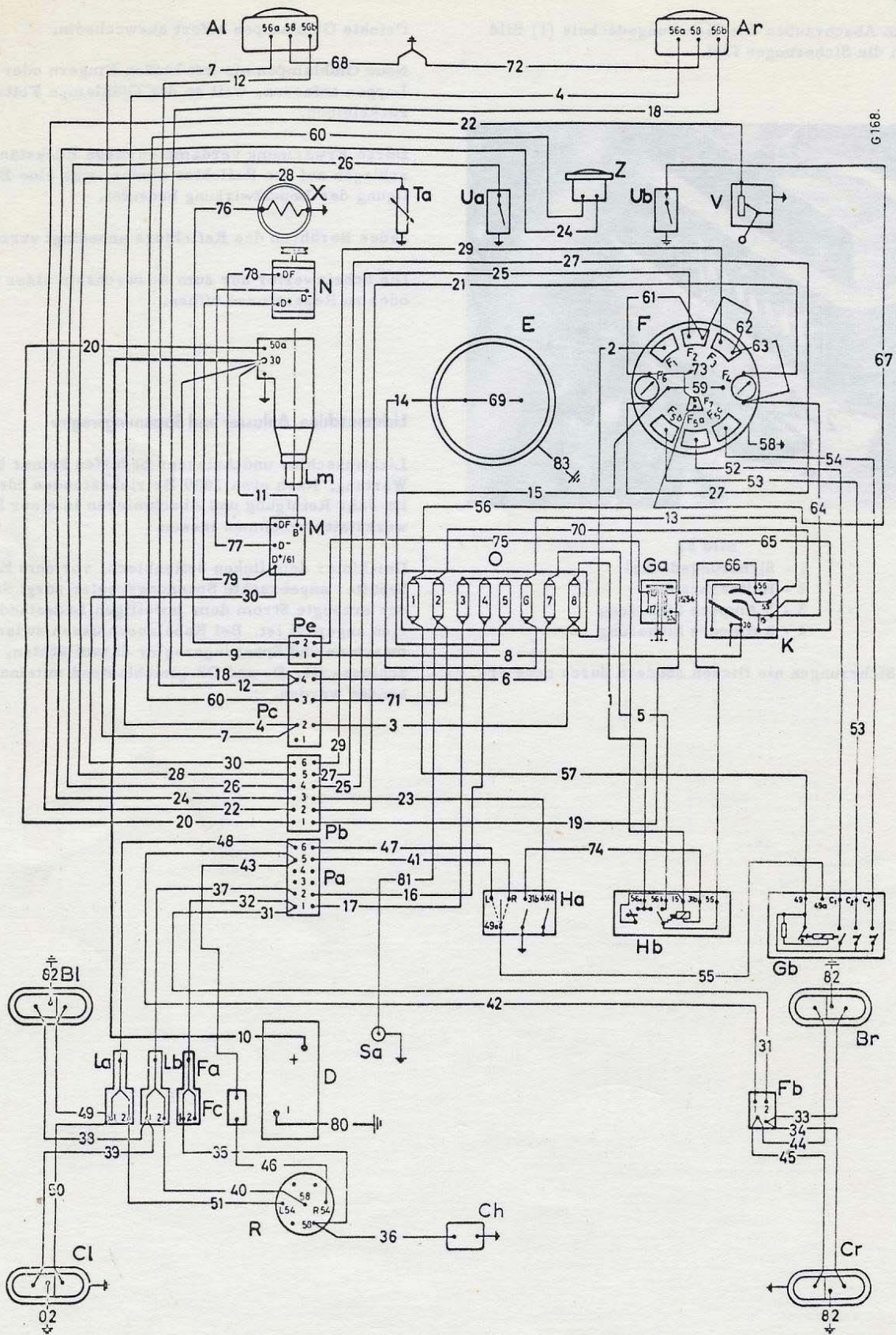
* Schaltschema für Schlepper mit Geschwindigkeiten bis 20 km/std.
